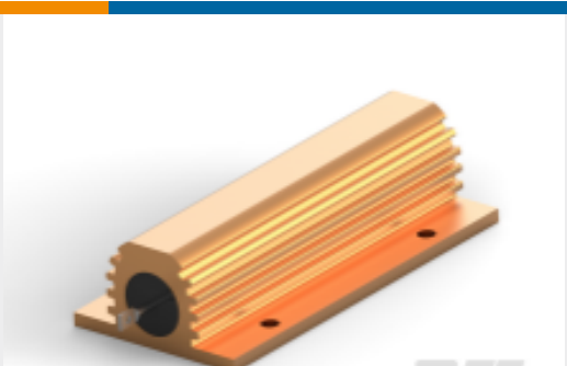
TE 产品编号1630027-5 功率电阻器：铝壳体，HSC
