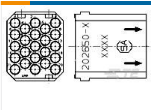
TE 产品编号202650-4 PIN MODULE, 23 POSN, G-SERIES
