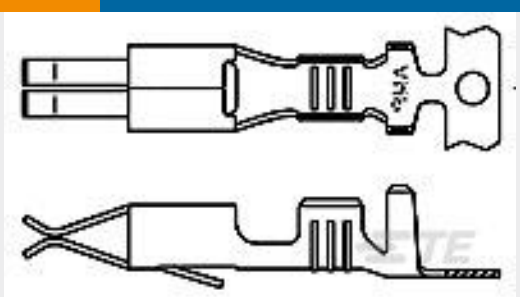
TE 产品编号770520-3 AMPSEAL 端子
