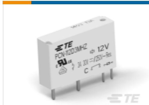
TE 产品编号1721081-4 PCN 3A/5A 纤薄 PCB 继电器 3VDC
