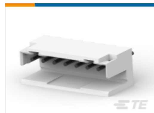
TE 产品编号1-292173-9 AMP 通用终端接头
