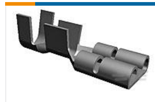
TE 产品编号100570-2 250 FASTON,REC.,14-17AWG,TPBR
