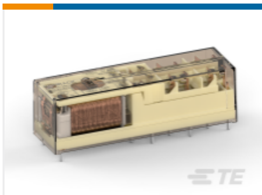
TE 产品编号1415015-1 增强绝缘强制导向继电器
