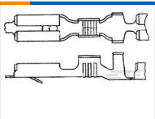
TE 产品编号170042-2 FF 110 REC 20-16AWG TPBR
