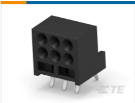
TE 产品编号1376962-1 FAN MOTOR CONN HDR ASSY T/E
