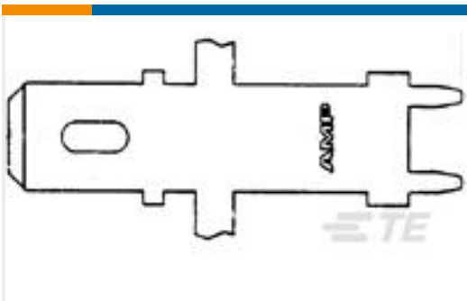
TE 产品编号63950-1 FASTON 250 PCB TAB BR
