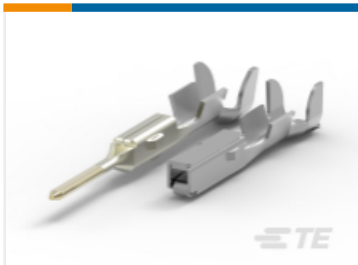
TE 产品编号173631-2 MULTILOCK，母端和公端
