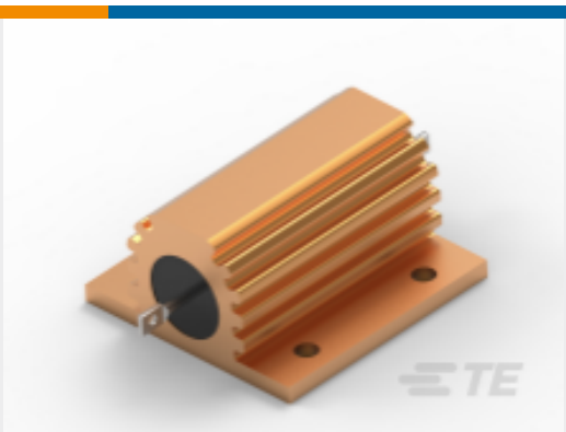
TE 产品编号1630186-1 功率电阻器：铝壳体，HSA
