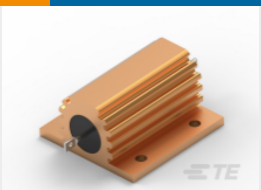
TE 产品编号4-1630012-1 功率电阻器：铝壳体，HSA
