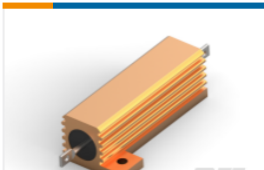
TE 产品编号1676814-7 功率电阻器：铝壳体，HSA
