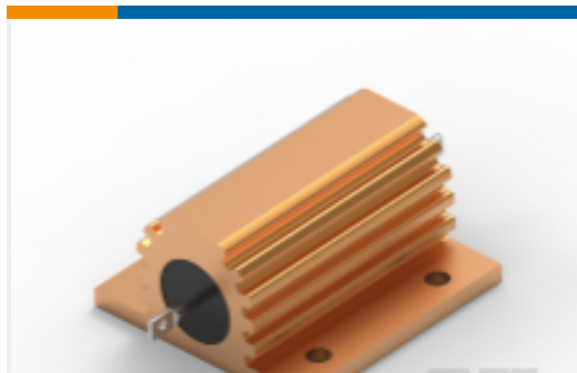
TE 产品编号1630019-4 功率电阻器：铝壳体，HSA
