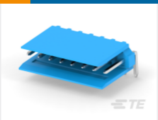
TE 产品编号281699-2 HE13/HE14 TH 接头，SRRA
