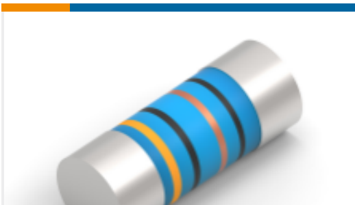
TE 产品编号2176315-6 MELF SMA_A 270R 0.1% 15PPM 0204 0.4W
