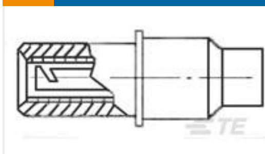
TE 产品编号517641-000 D-602-1113
