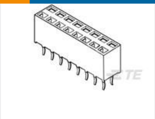
TE 产品编号1-215307-4 2X14P HV100 REC CON. TE, 7.0MM
