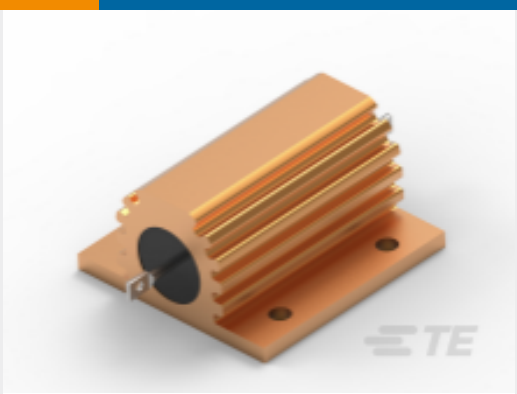
TE 产品编号1-1630019-9 功率电阻器：铝壳体，HSA
