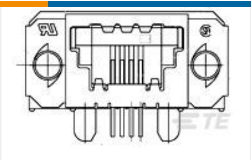
TE 产品编号1-1761185-3 8 SDL SE GRND RCPT ASSY
