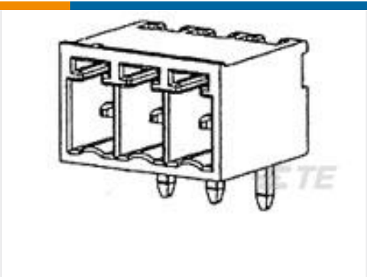
TE 产品编号1-284512-0 10 POS TERMI-BLOK HDR 900 POLA
