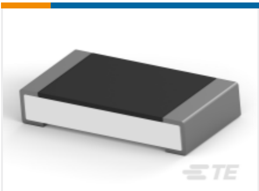
TE 产品编号1-2176392-4 RQ 1206 182K 0.1% 10PPM 5K RL
