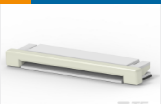
TE 产品编号2041215-1 .5mm FPC 连接器
