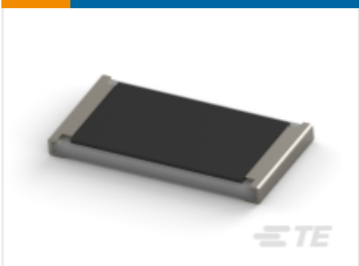
TE 产品编号1-2176070-0 SMD 功率电阻器：2 瓦特，3521 系列
