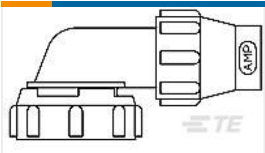
TE 产品编号213982-1 R/A STRN RELIEF KIT,SZ 13,CPC
