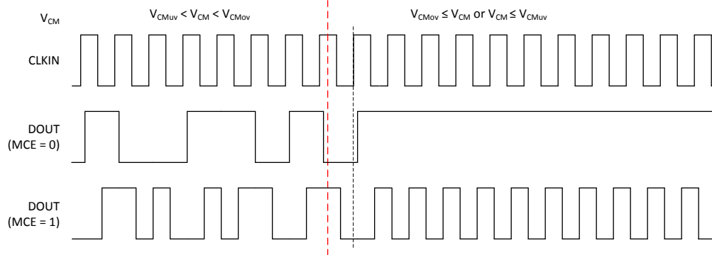
图 44. Fail-Safe Output of the AMC1035-Q1
