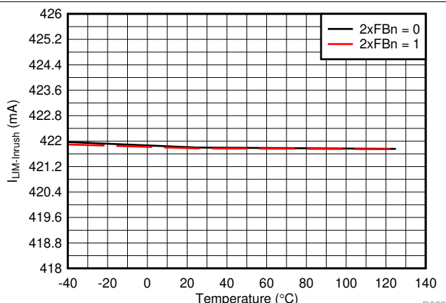
图 21. 浪涌电流限制与温度间的关系
