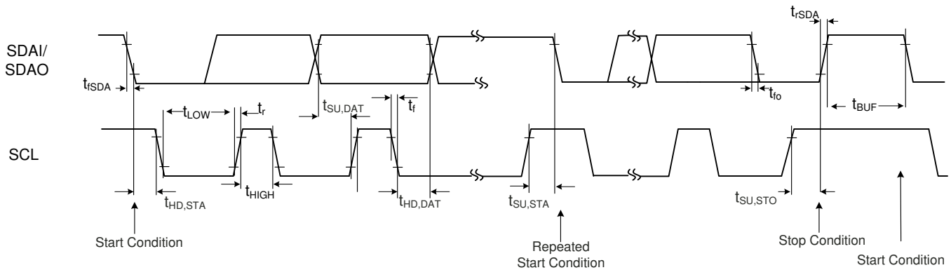
图 29. I²C 时序
