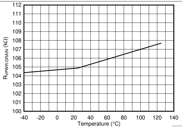
图 25. R_{\text{OFF}} (VPWR 至 DRAIN) 与温度间的关系
