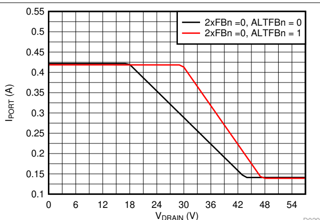
图 27. 1x 模式 ( 2\text{xFBn} = 0 ) 电流折返与漏极电压间的关系
