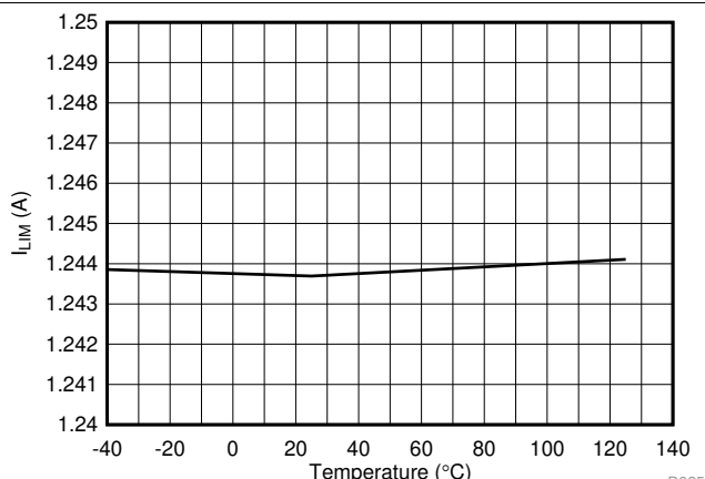
图 23. 2x 模式 ( 2x\text{FBn} = 1 ) 电流限制与温度间的关系
