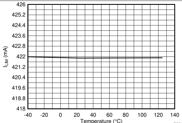
图 22. 1x 模式 ( 2x\text{FBn} = 0 ) 电流限制与温度间的关系
