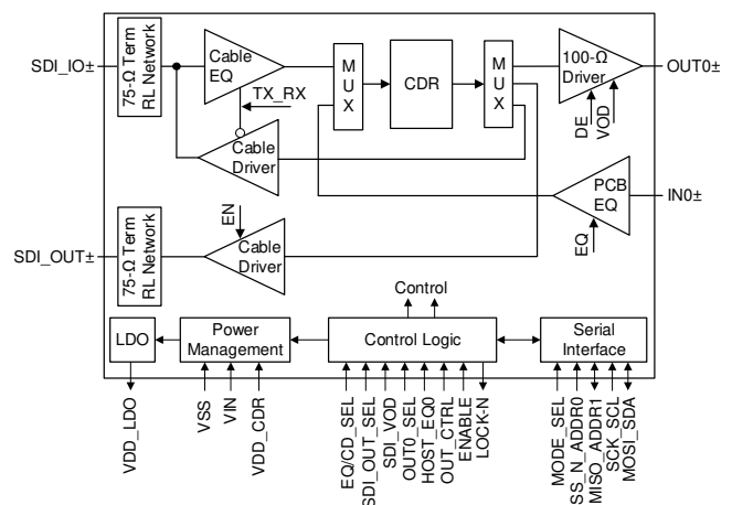
简化方框图
