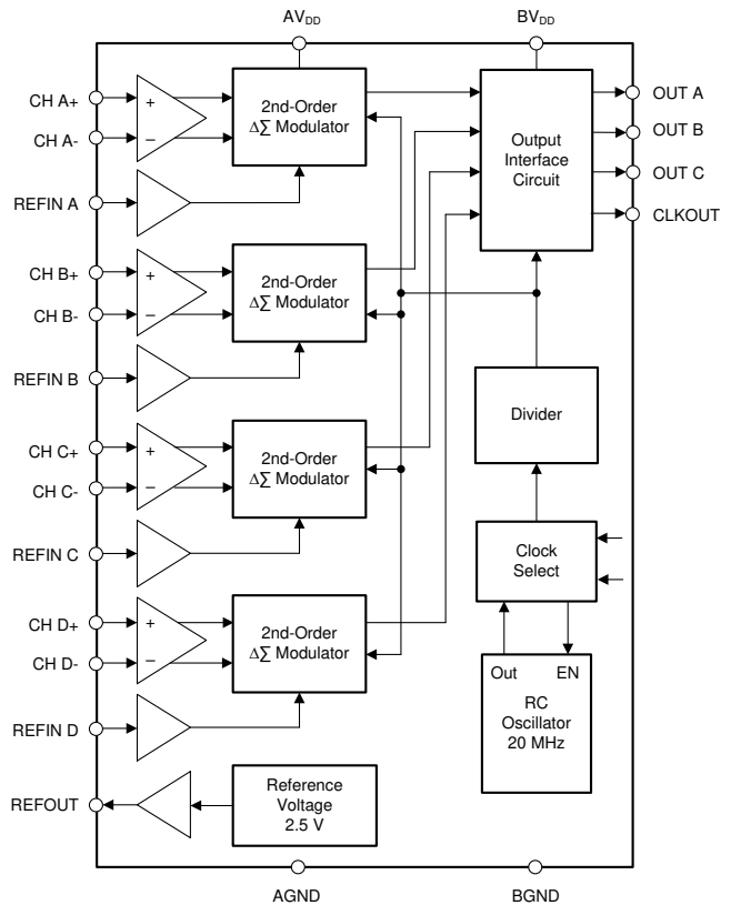
功能方框图
