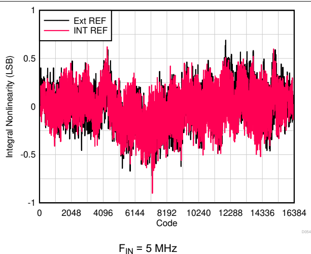
图 6-18. INL vs Code
