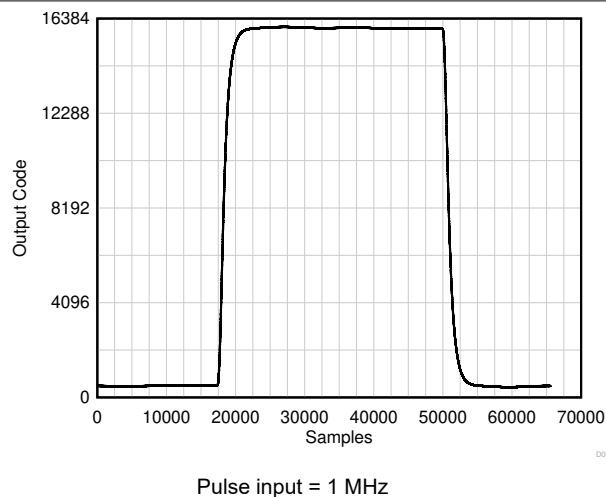
图 6-21. Pulse Response
