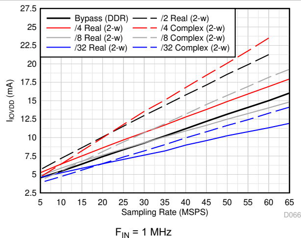
图 6-23. I_{IOVDD} Current vs Decimation
