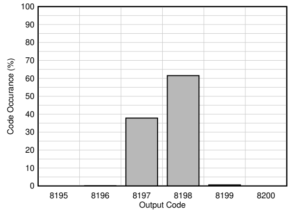
图 6-20. DC Histogram
