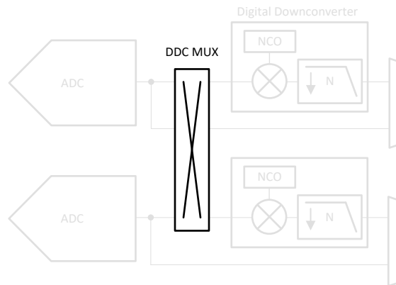
图 8-19. DDC MUX
