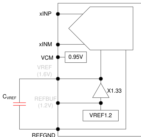
图 8-15. Internal reference
