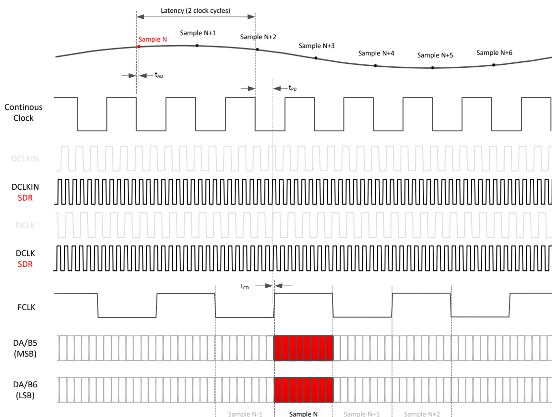
图 8-38. SDR Output Clocking
