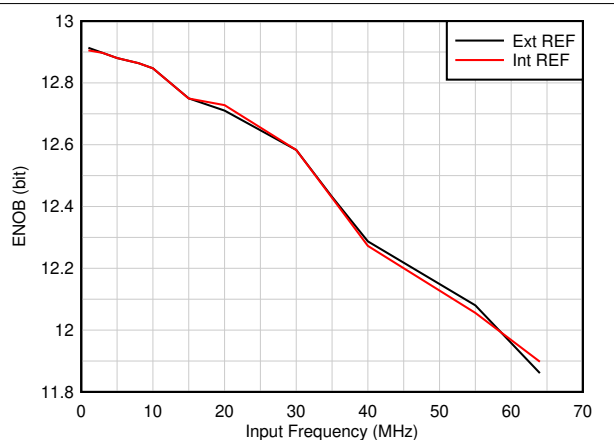
图 6-10. ENOB vs Input Frequency
