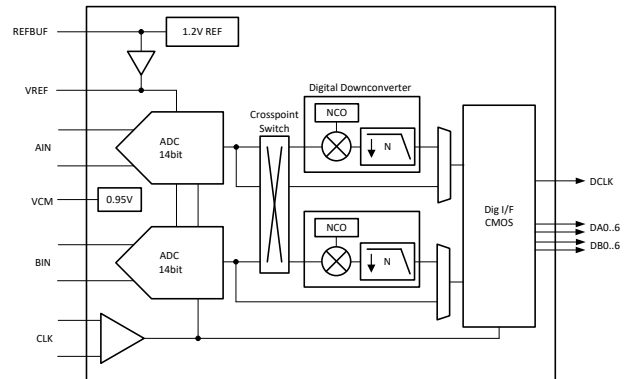
ADC364x 方框图
