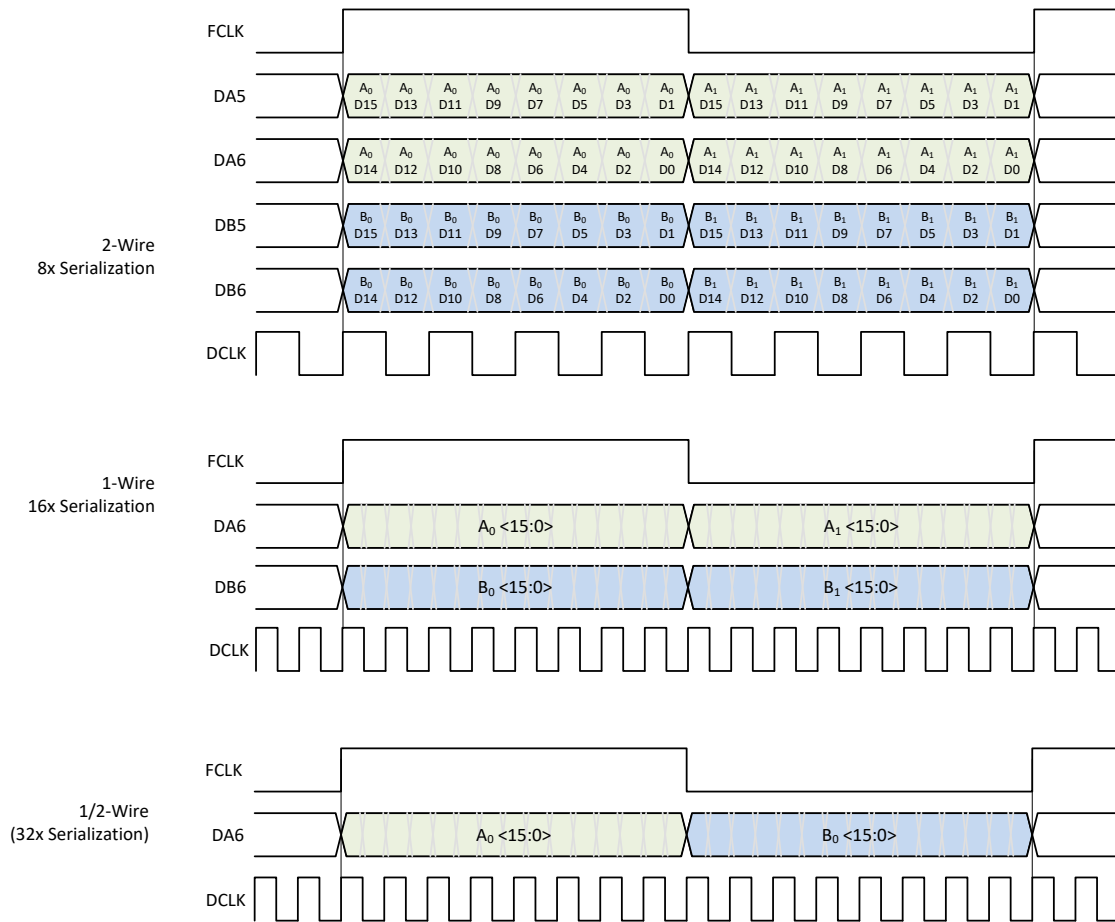
图 8-37. Output Data Format in Real Decimation
