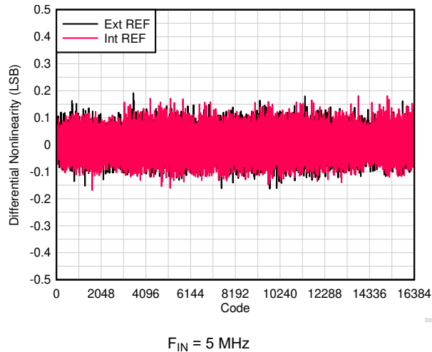
图 6-19. DNL vs Code
