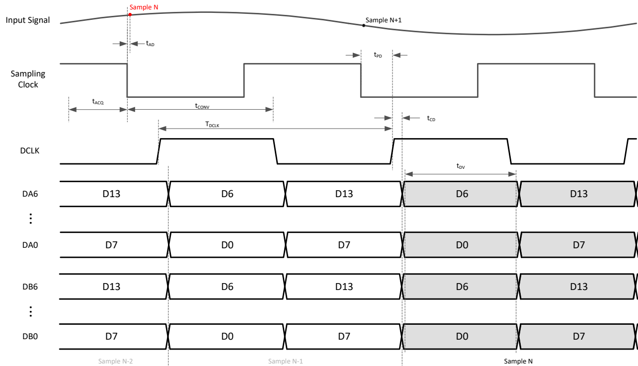
图 7-1. Timing diagram: DDR CMOS
