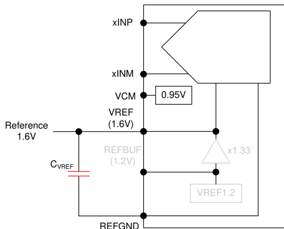
图 8-16. External 1.6V reference
