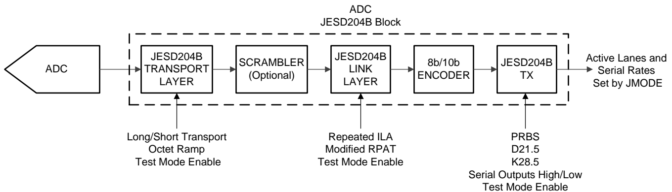
图 94. Test Mode Insertion Points
