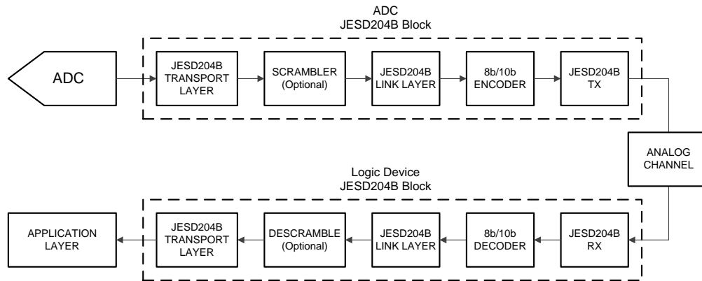
图 91. Simplified JESD204B Interface Diagram
