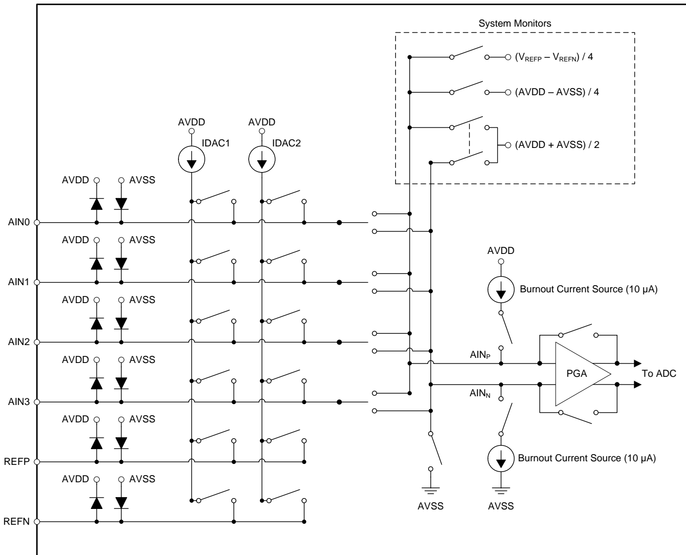
图 42. Analog Input Multiplexer
