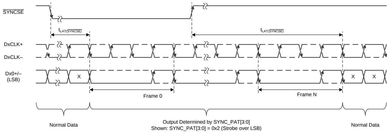
图 8. SYNCSE Timing Diagram
