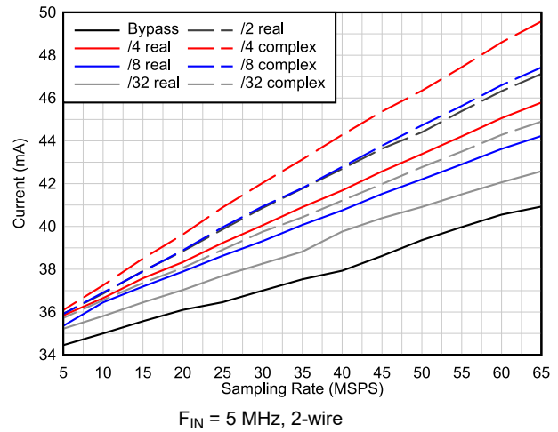
图 6-24. Current vs Decimation
