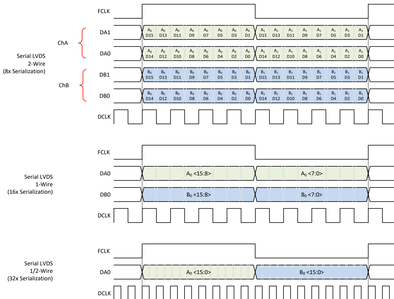
图 8-37. Output Data Format in Real Decimation
