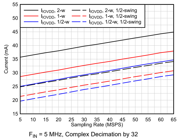
图 6-25. Current vs Output Interface
