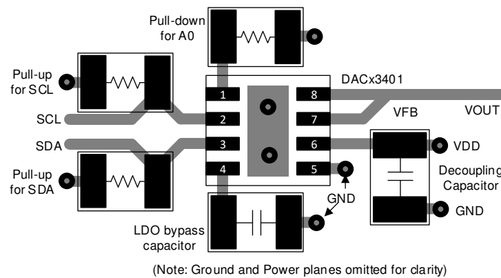
图 75. Layout Example
