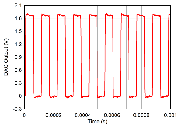
图 74. Pulse Frequency
