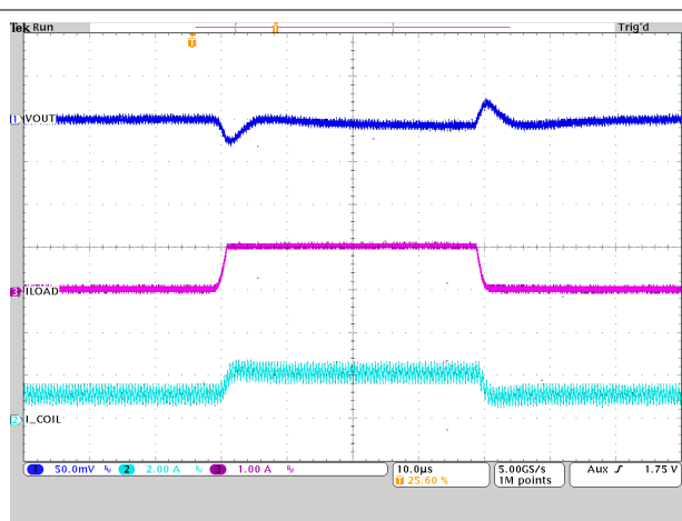
图 9-46. Load Transient
