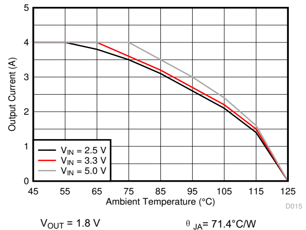
图 9-30. Thermal Derating
