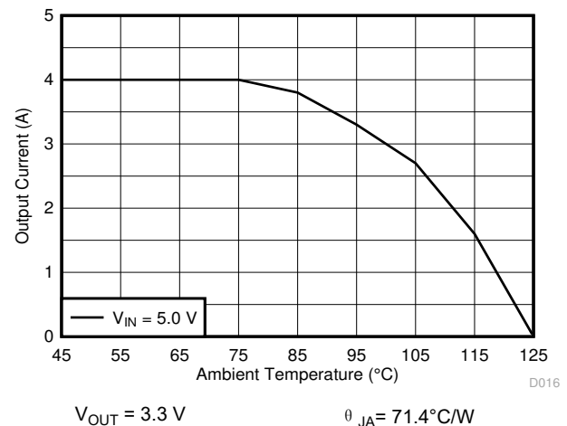
图 9-32. Thermal Derating
