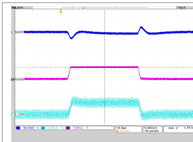
图 9-45. Load Transient
