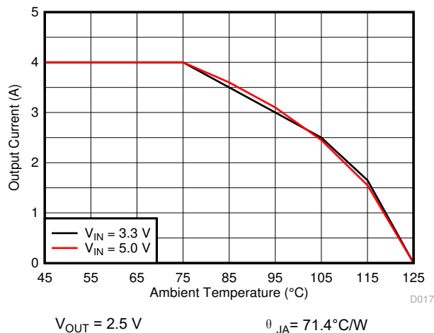
图 9-31. Thermal Derating
