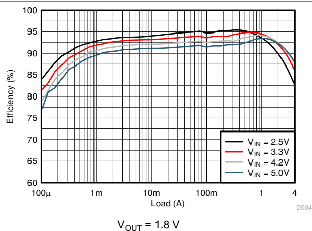
图 9-11. Efficiency
