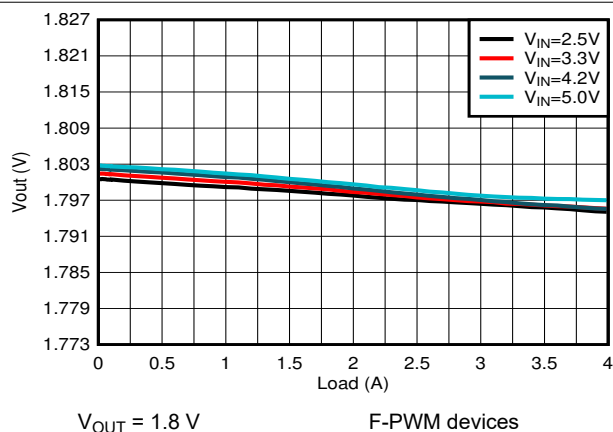
图 9-14. Load Regulation
