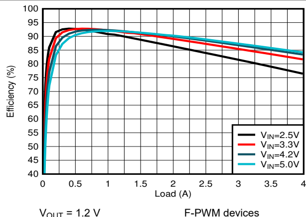
图 9-9. PWM Efficiency
