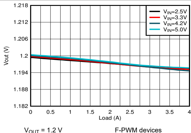
图 9-10. Load Regulation
