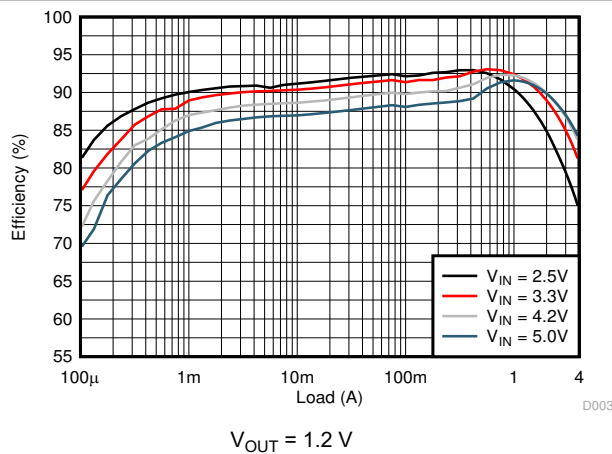
图 9-7. Efficiency
