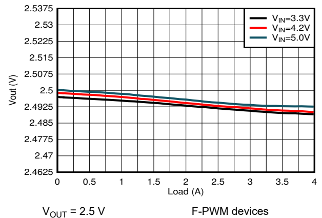
图 9-18. Load Regulation
