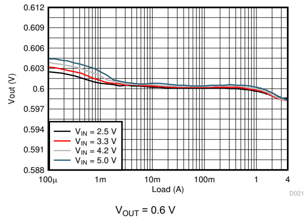
图 9-4. Load Regulation
