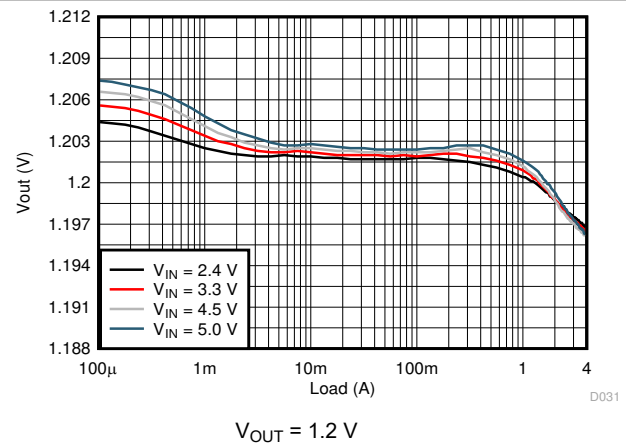
图 9-8. Load Regulation
