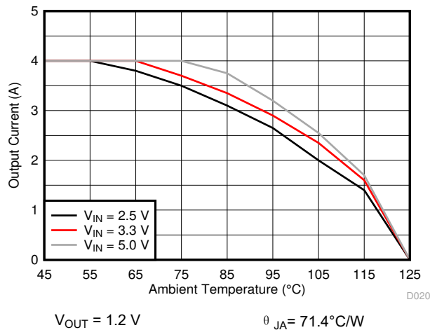
图 9-29. Thermal Derating
