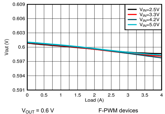
图 9-6. Load Regulation
