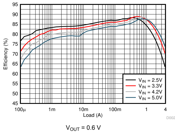
图 9-3. Efficiency
