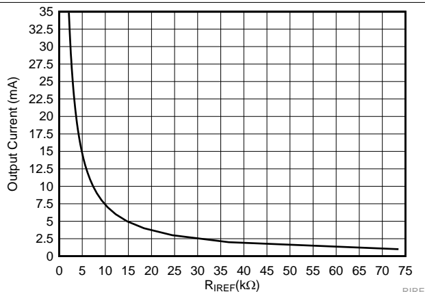
图 2. I_{OUT} Target vs R_{REF}
