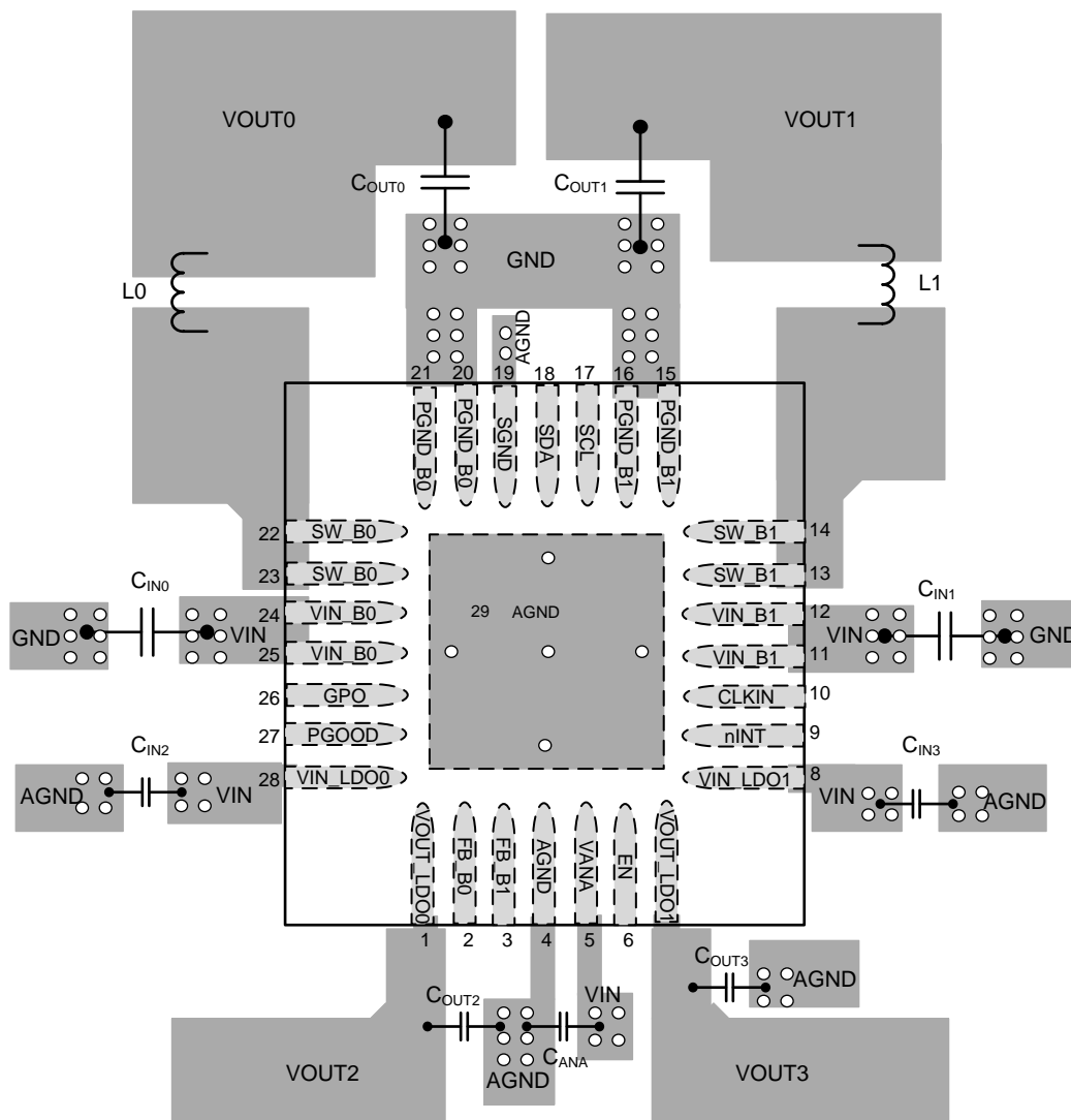
图 55. LP87332A-Q1 Board Layout
