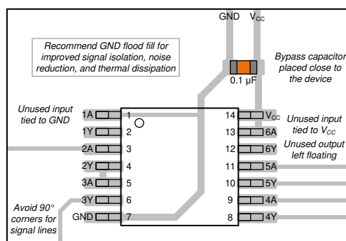
图 11. Example layout for the SN74HCS14-Q1
