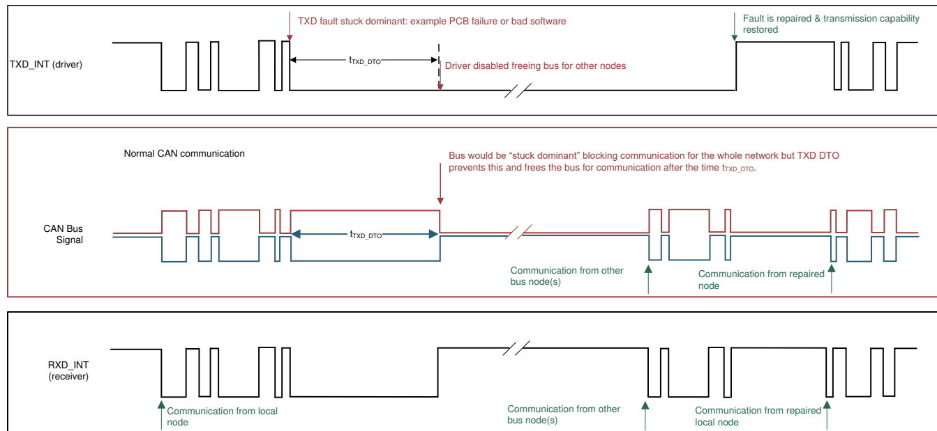
图 25. Example timing diagram with TXD_INT DTO
