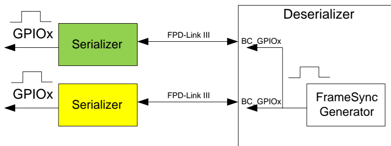
图 8. Internal FrameSync
