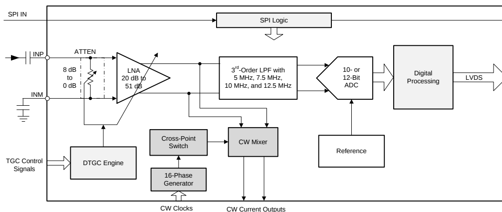
简化框图
