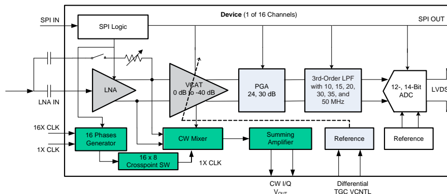
简化框图
