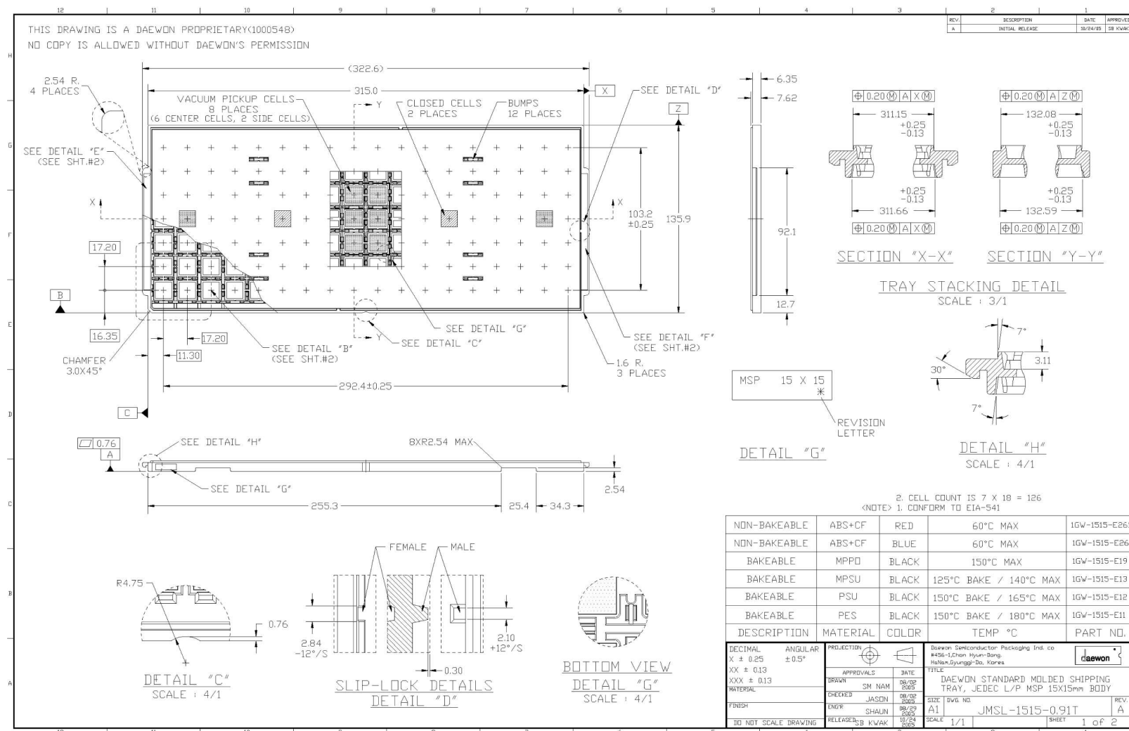
图 169. 托盘图, 第 1 节
