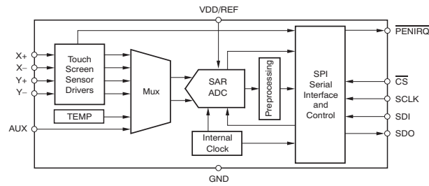
图 1. 方框图
