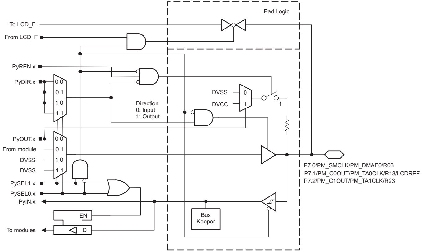
图 6-10. P7.0, P7.1 and P7.2 Port Schematic
