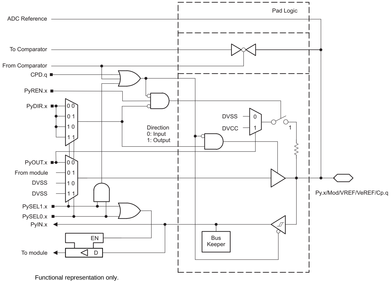
图 6-14. Py.x/Mod/VREF/VeREF/Cp.q Port Schematic
