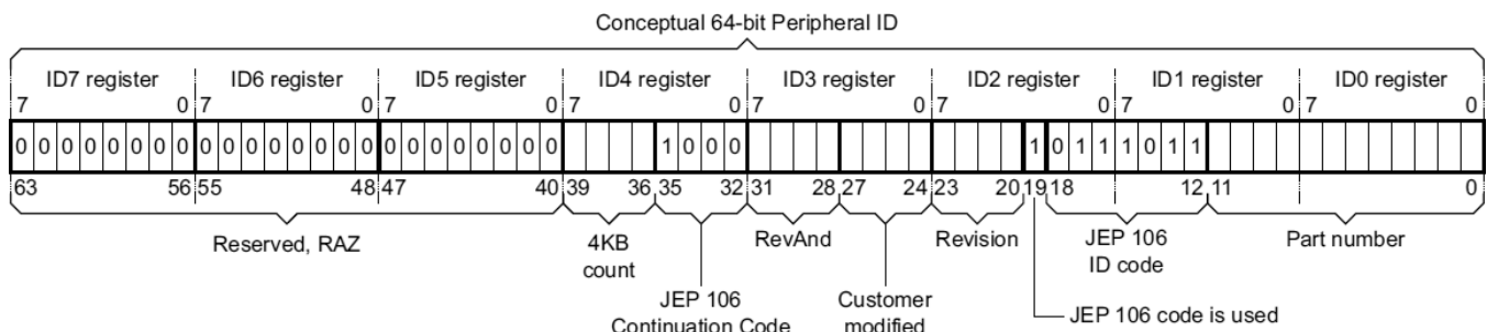
图 6-24. Arm Cortex-M4 Peripheral ID Register Description
