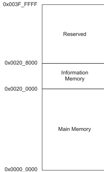
图 6-5. Flash Memory Map
