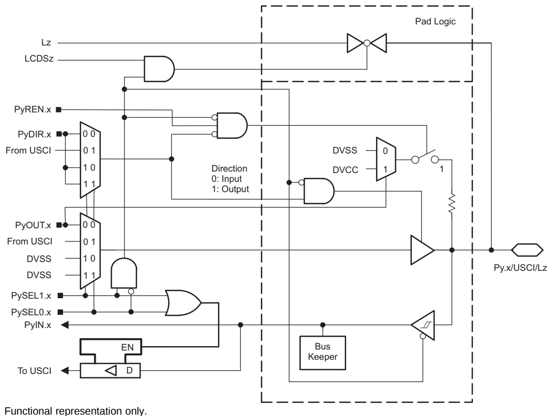
图 6-8. Py.x/USCI/Lz Port Schematic
