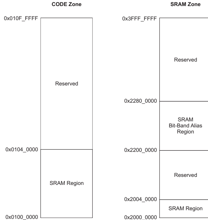
图 6-6. SRAM Map
