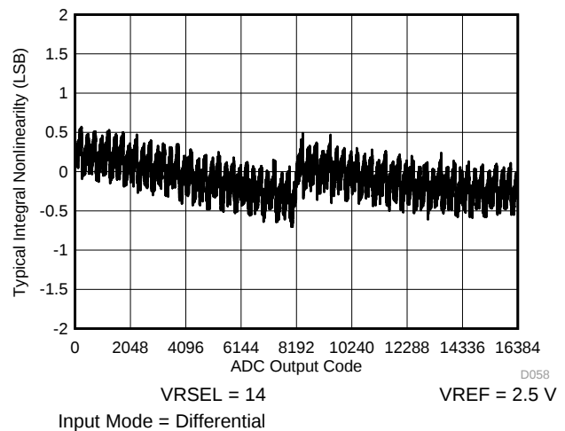
图 5-38. INL vs ADC Output Code
