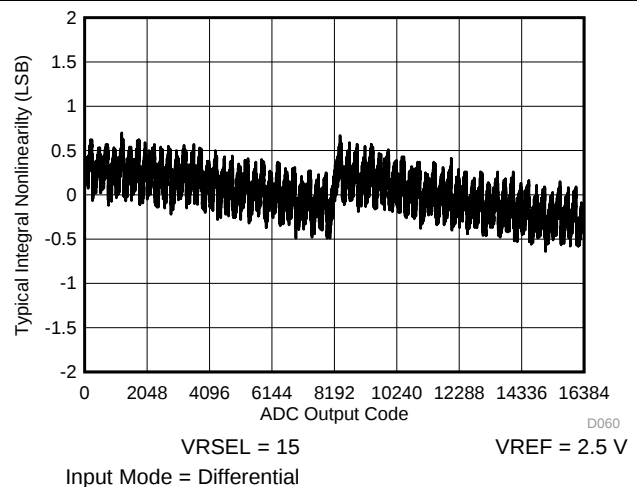
图 5-40. INL vs ADC Output Code
