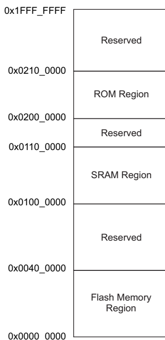
图 6-2. Code Zone Memory Map
