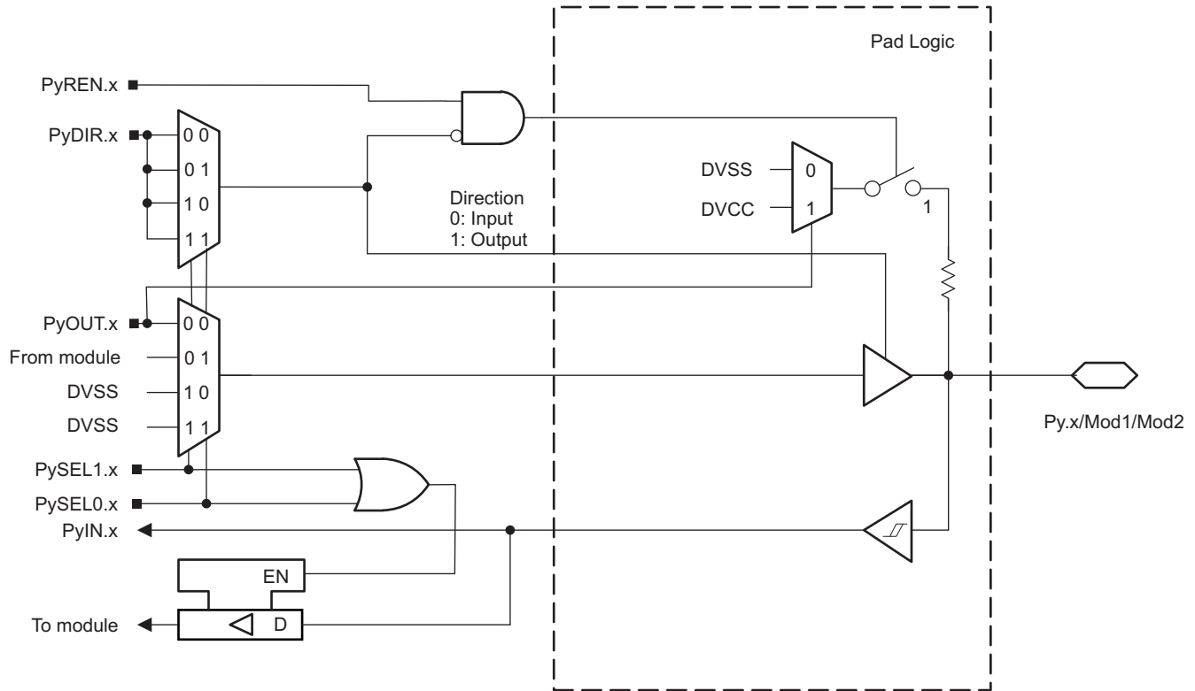
图 6-11. P7.3 Port Schematic
