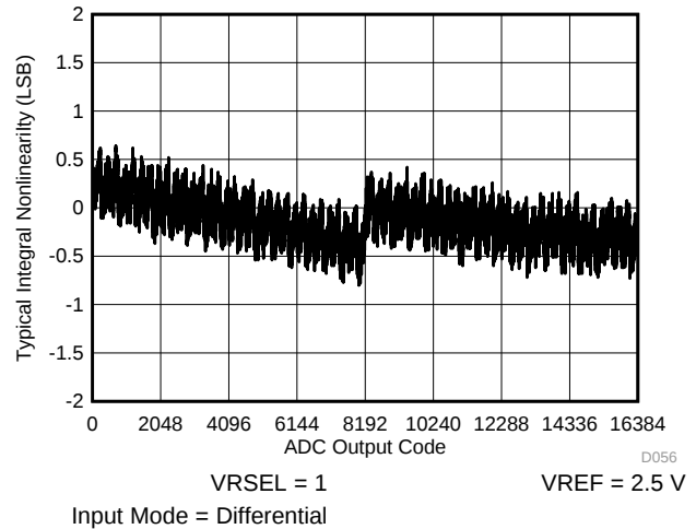
图 5-36. INL vs ADC Output Code
