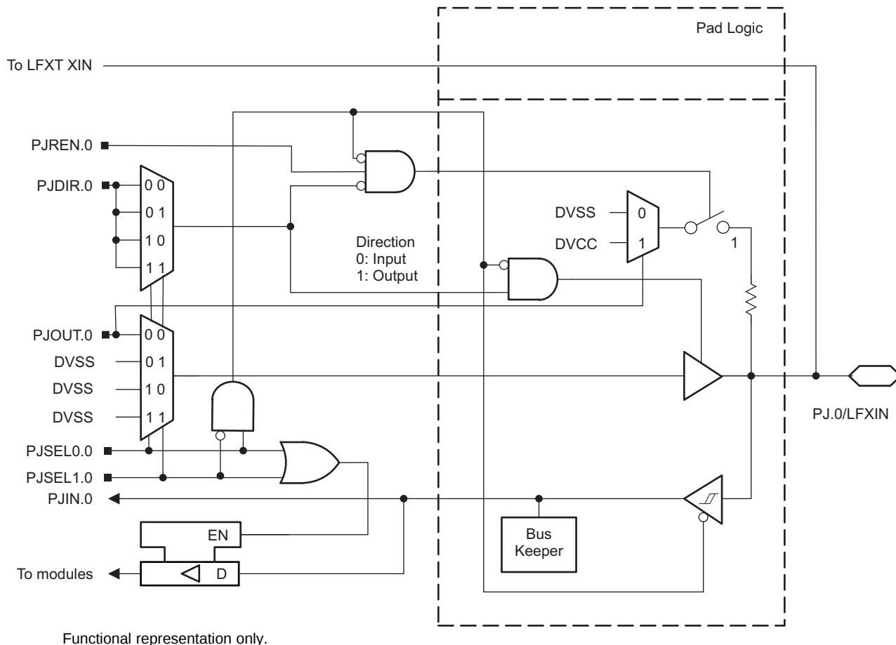
图 6-20. Port PJ (PJ.0) Port Schematic
