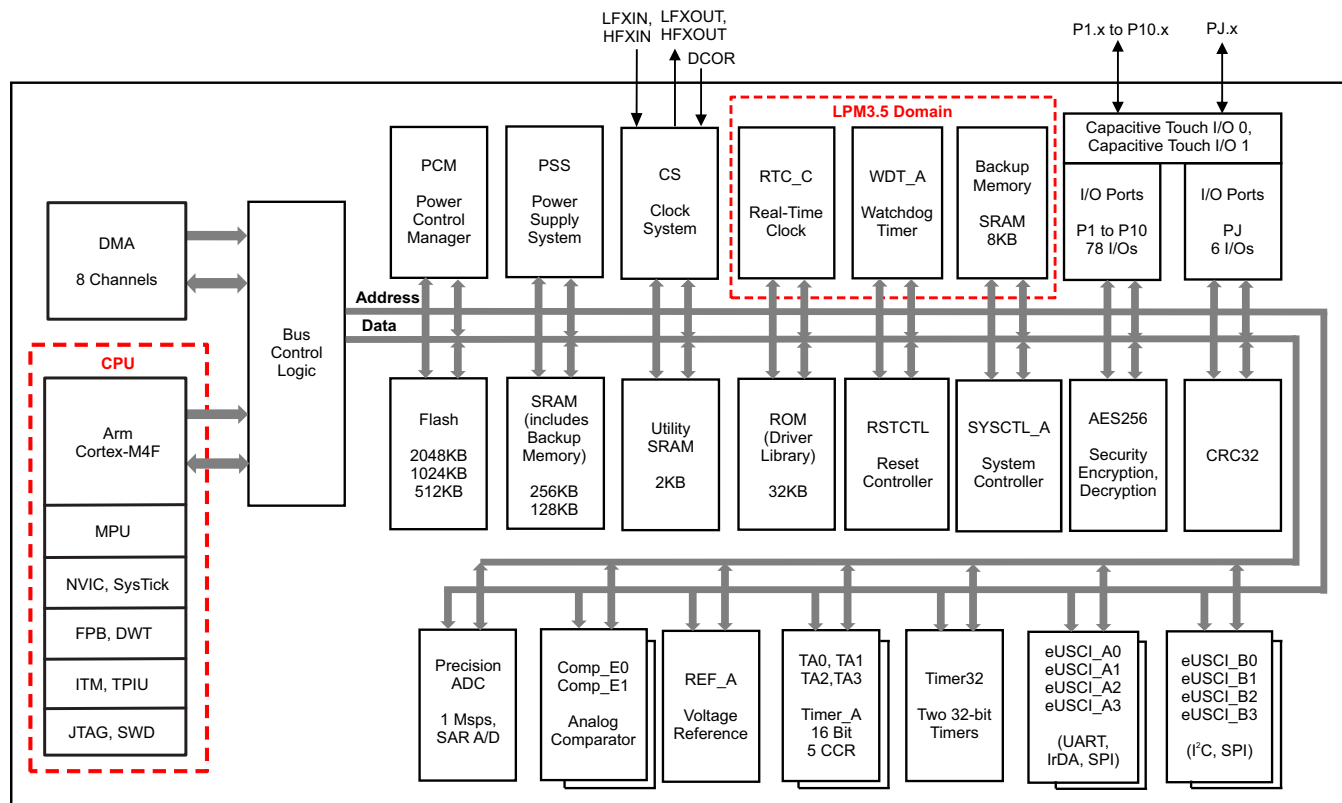
图 1-2. MSP432P401x 功能方框图
