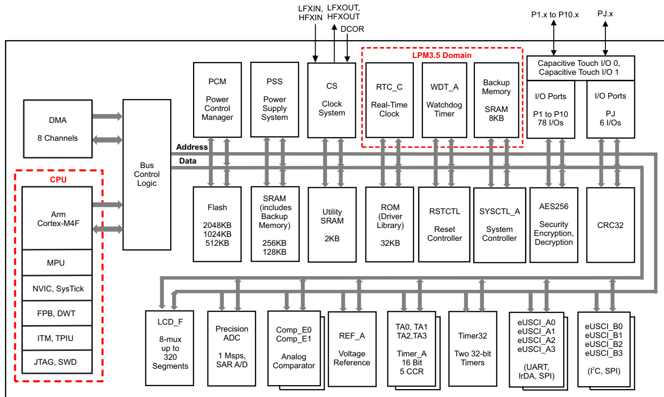
图 1-1. MSP432P411x 功能方框图
