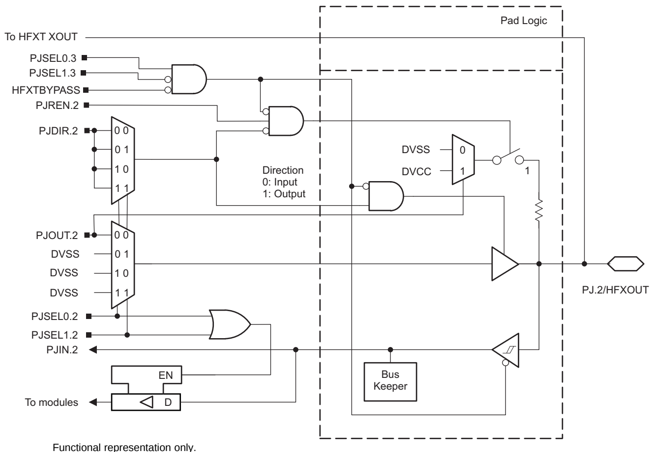
图 6-22. Port PJ (PJ.2) Port Schematic
