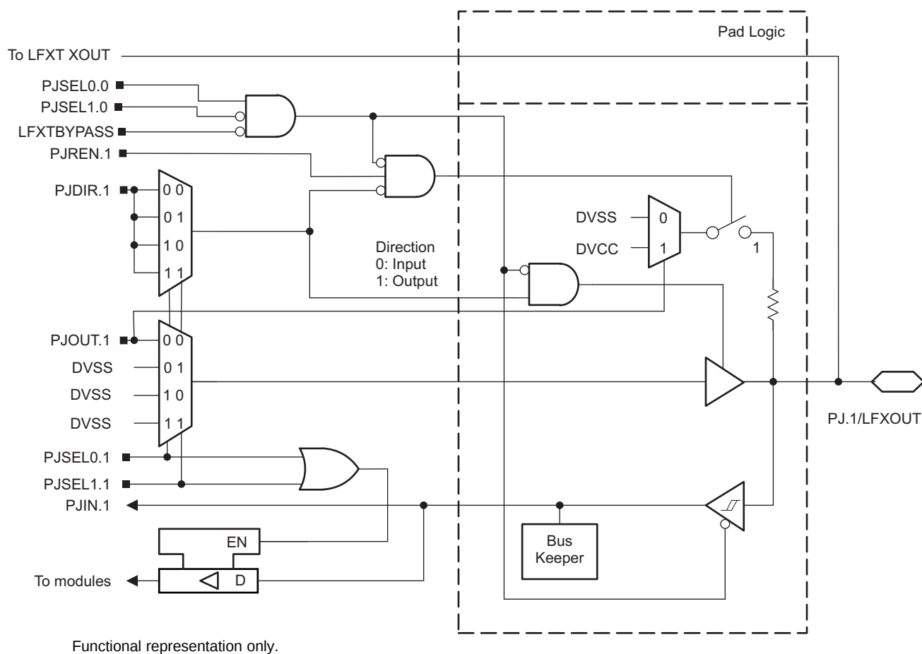
图 6-21. Port PJ (PJ.1) Port Schematic
