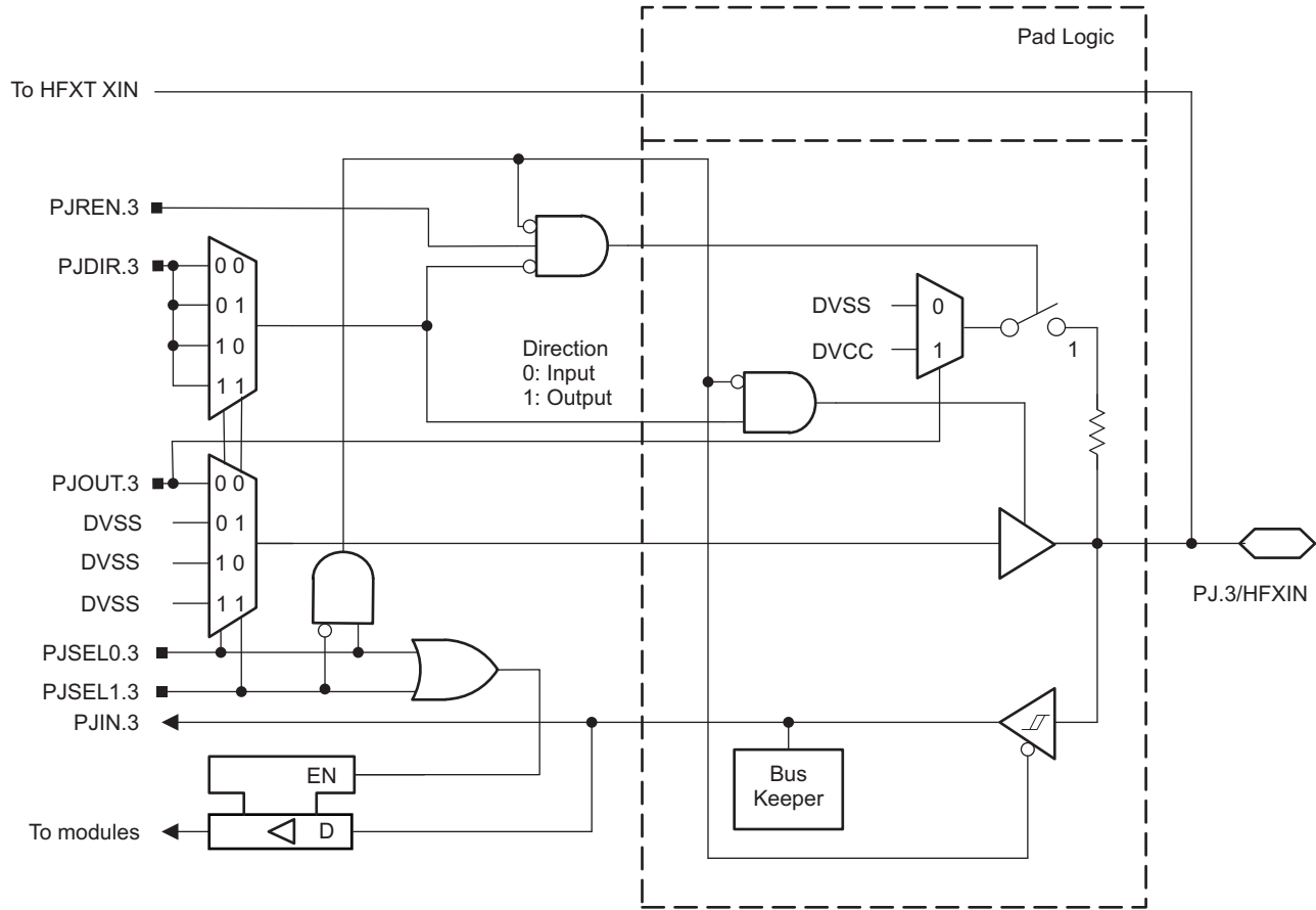
图 6-23. Port PJ (PJ.3) Port Schematic
