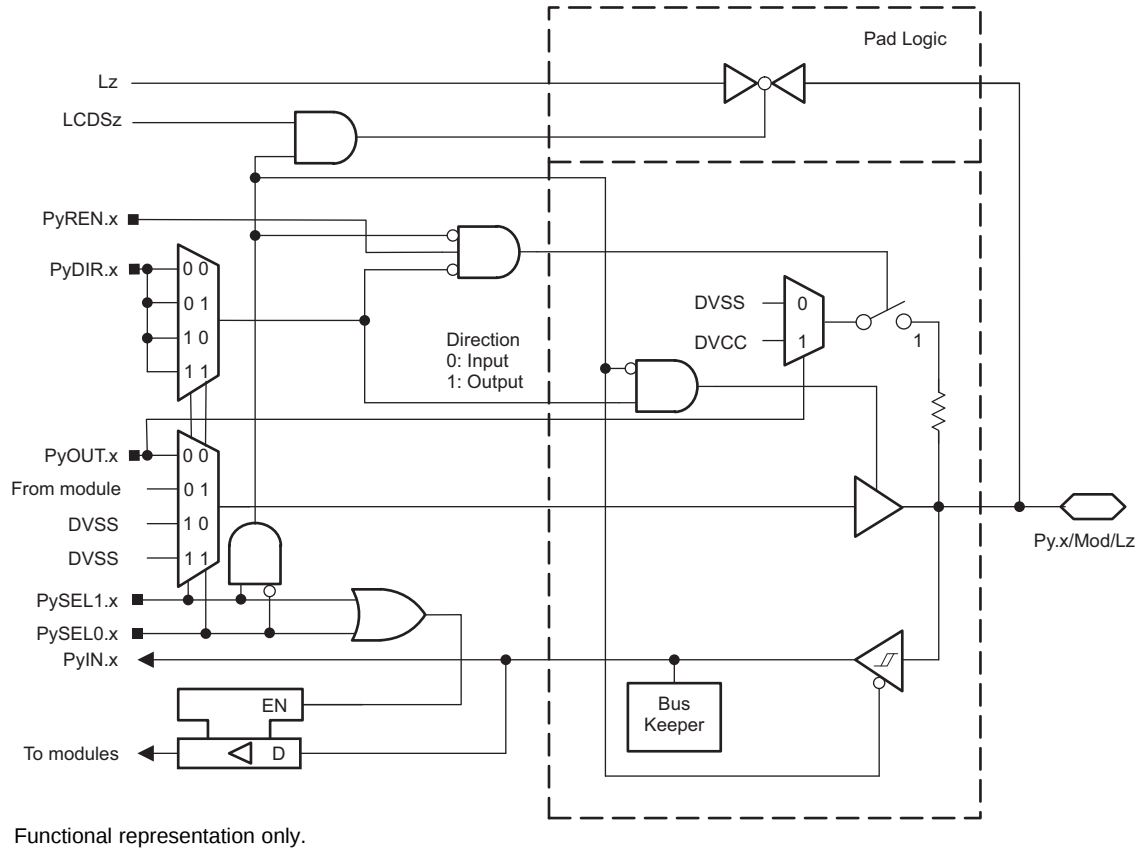
图 6-9. Py.x/Mod/Lz Port Schematic
