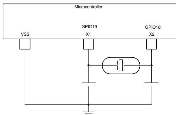
图 7-13. External Crystal
