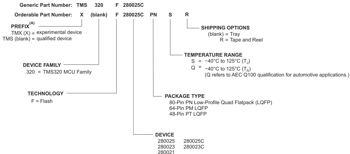
图 10-1. Device Nomenclature
