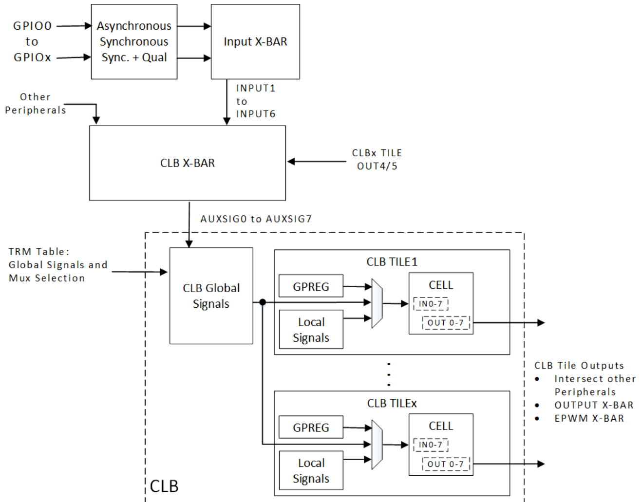
图 8-4. CLB Overview
