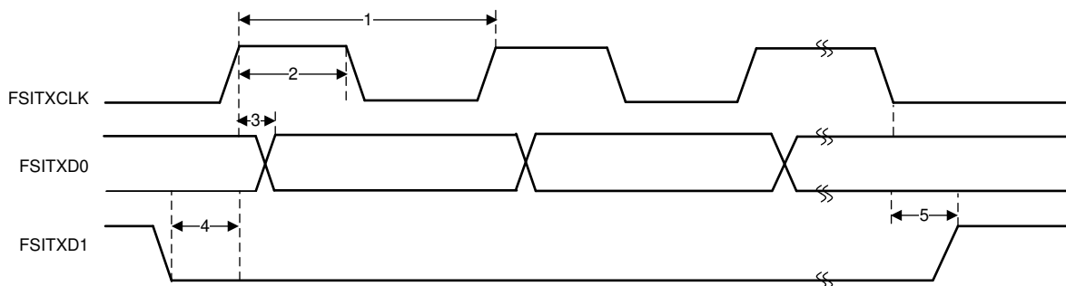
图 7-69. FSITX SPI Signaling Mode Timings
