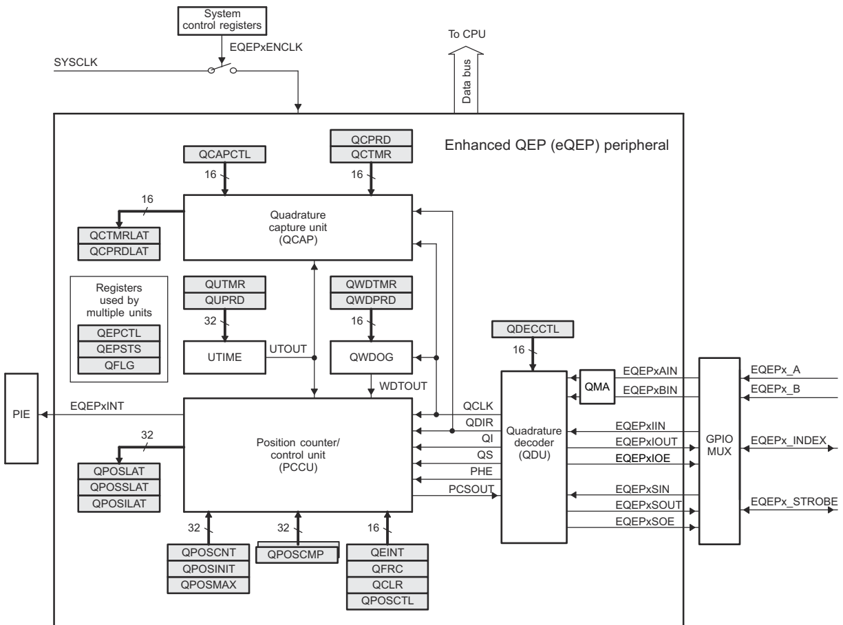
图 7-51. eQEP Block Diagram
