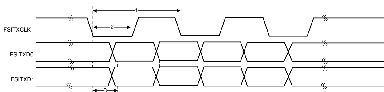
图 7-65. FSITX Timings
