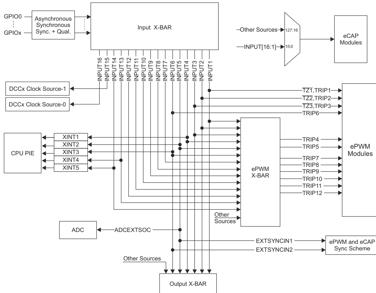
图 6-4. Input X-BAR
