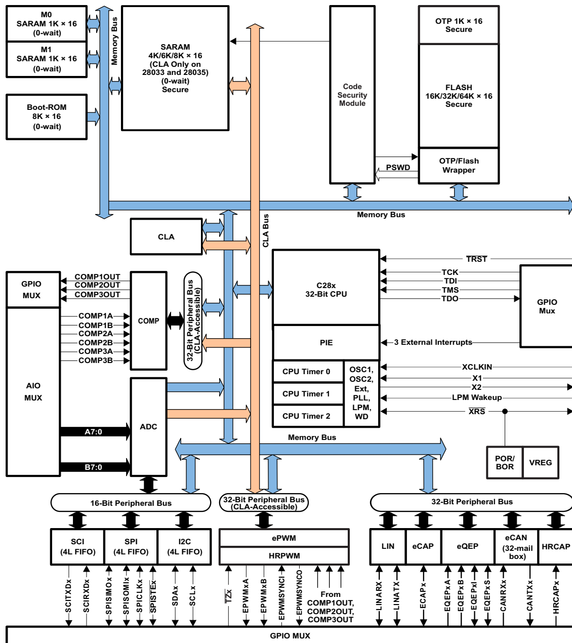
图 1-1. 功能方框图
