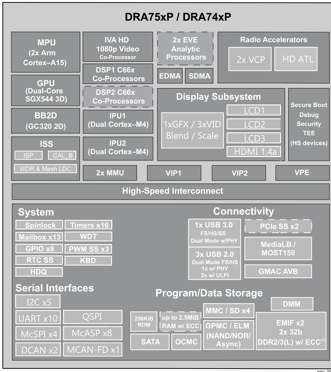
图 1-1. DRA75xP、DRA74xP 方框图
