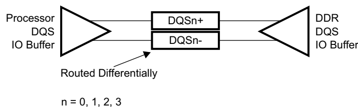
图 7-78. DQS Topology
