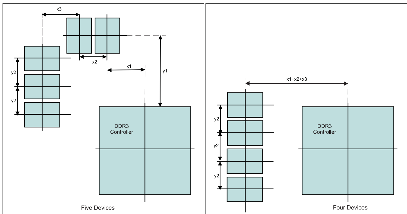
图 7-4. Placement Specifications
