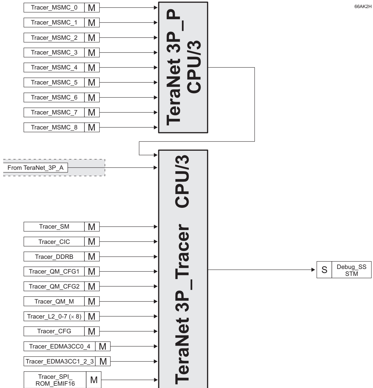
图 9-8. TeraNet 3P_Tracer
