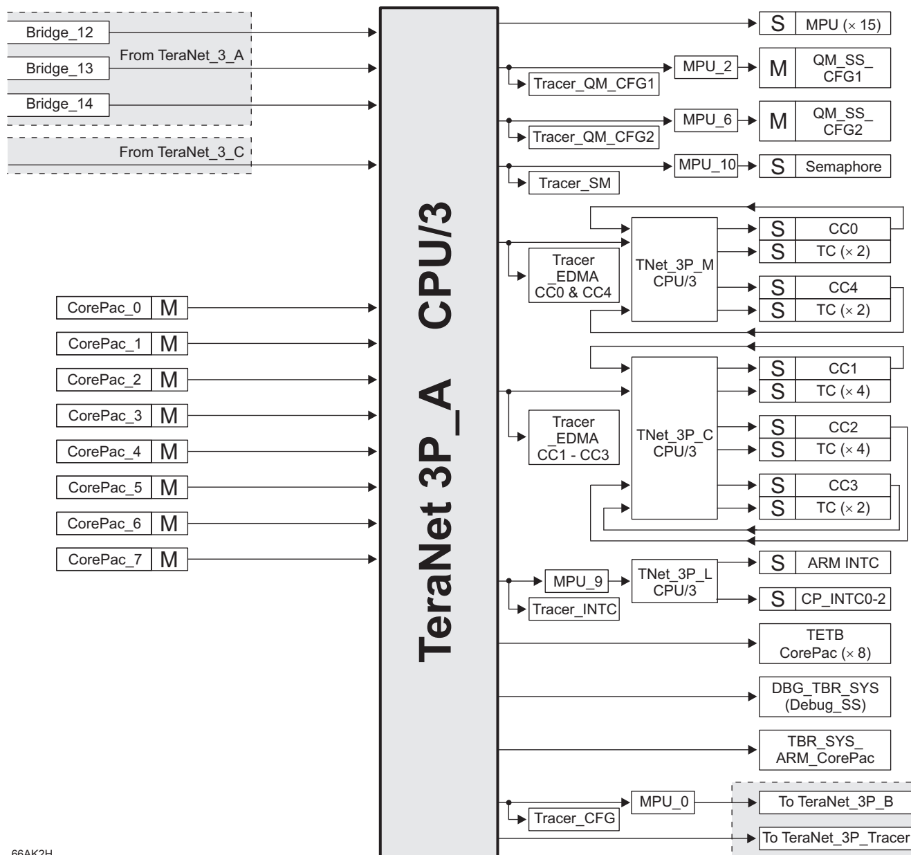
图 9-5. TeraNet 3P_A
