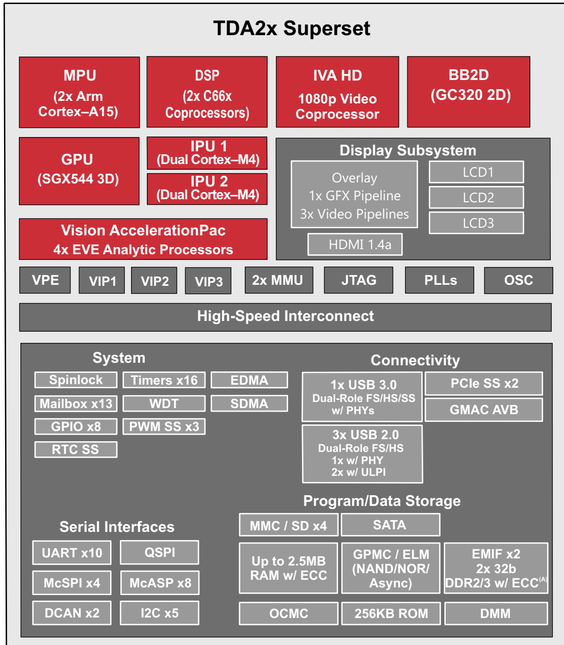
图 1-1. TDA2x 方框图
