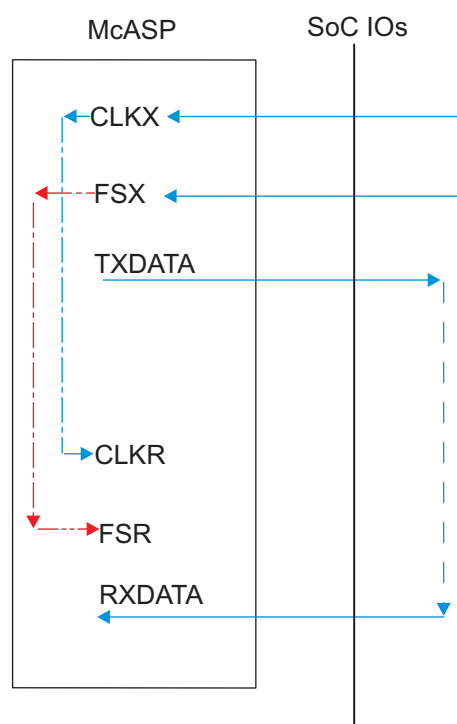
图 7-42. McASP1-8 CI-FI- – SYNC Mode
