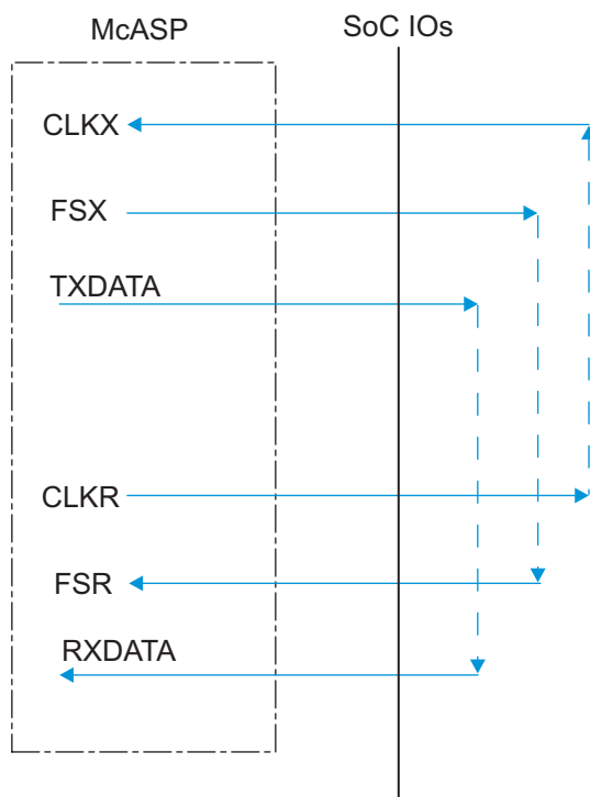
图 7-39. McASP1-8 CIOFOI – ASYNC Mode
