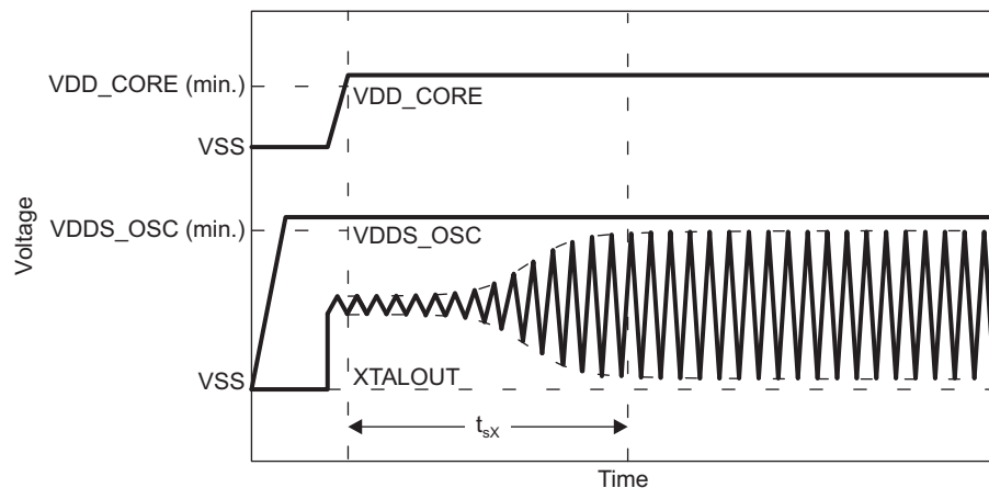
图 5-11. OSC0 Start-up Time
